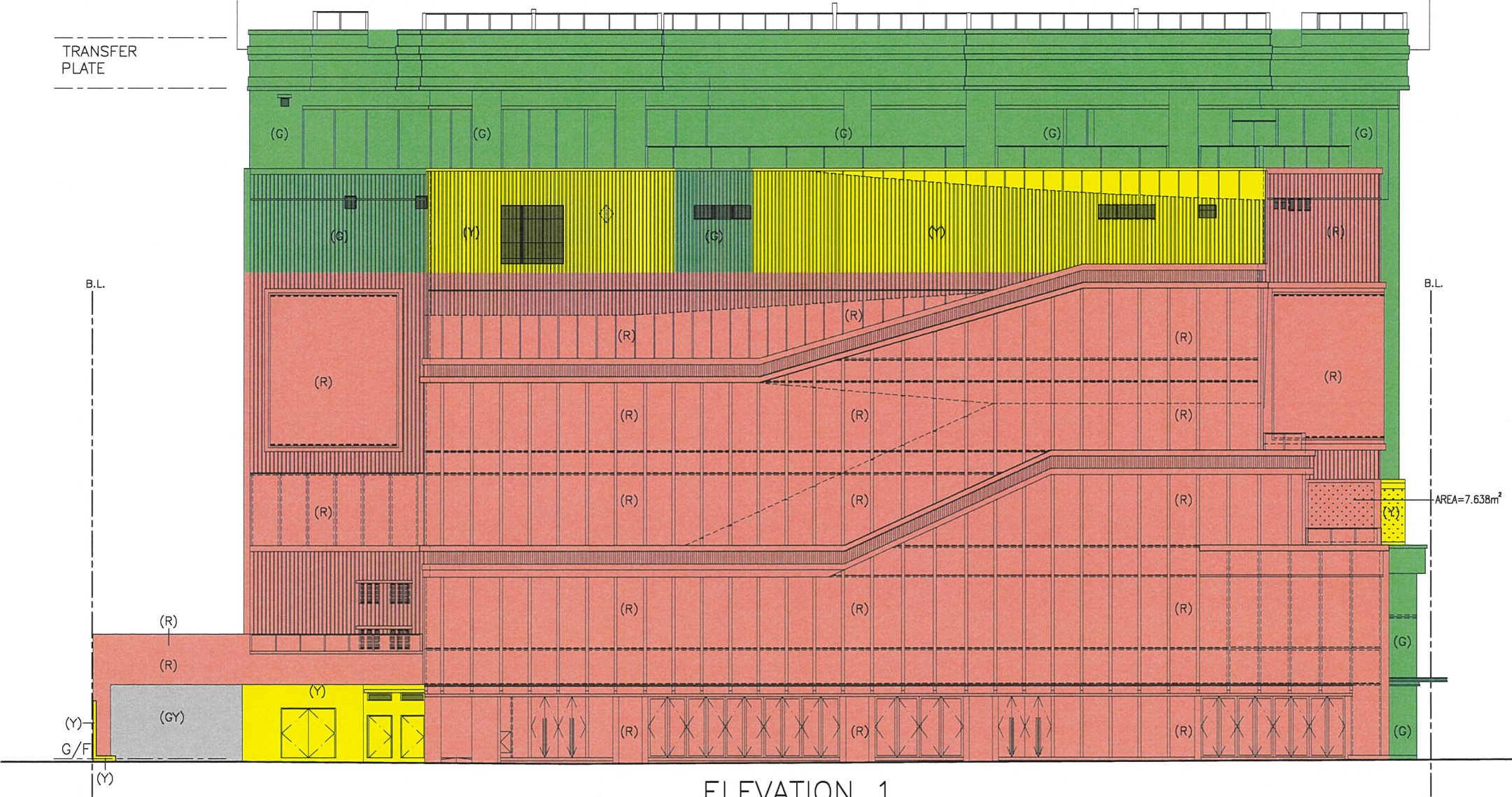
ELEVATION 1
