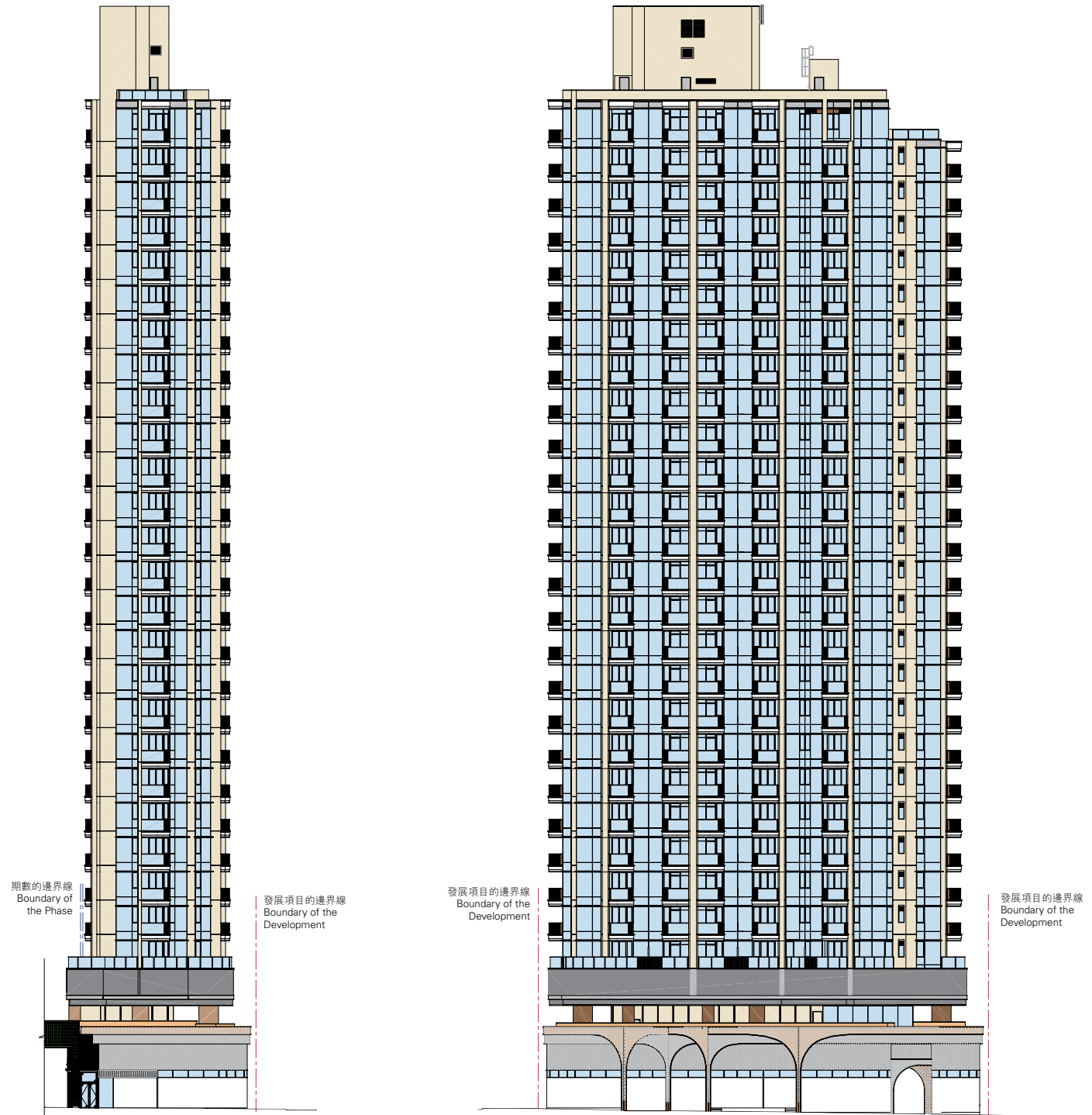
立面圖 3 ELEVATION PLAN 3
