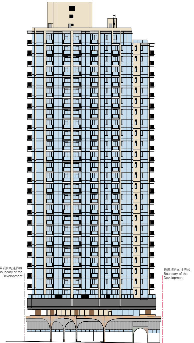
立面圖 4 ELEVATION PLAN 4
