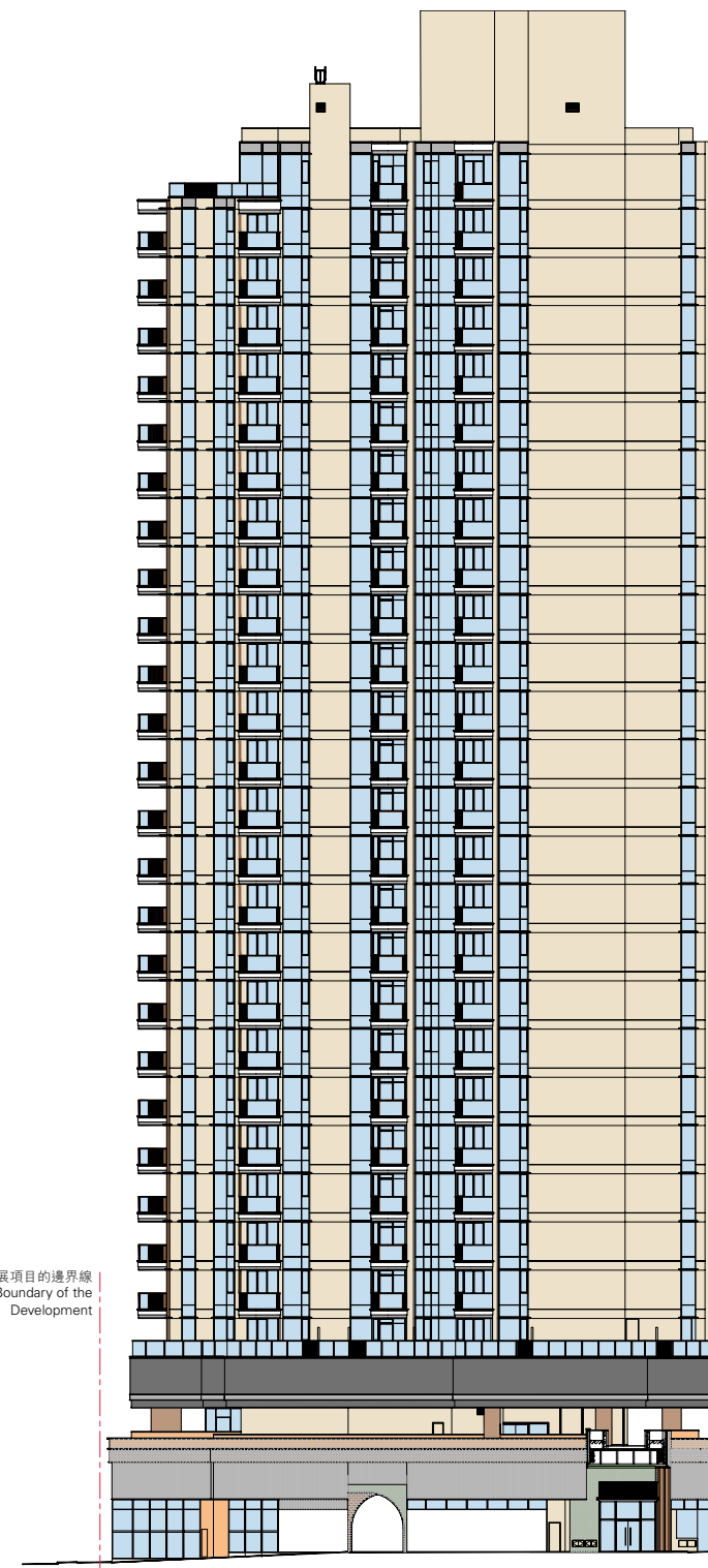
立面圖 2 ELEVATION PLAN 2
