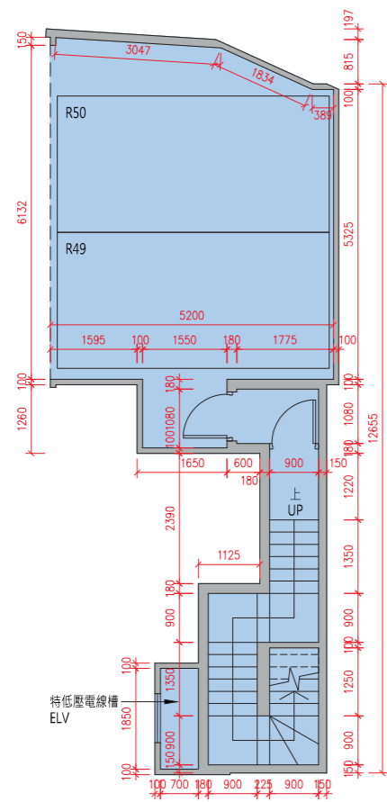
地庫1樓平面圖 B1/F Floor Plan
