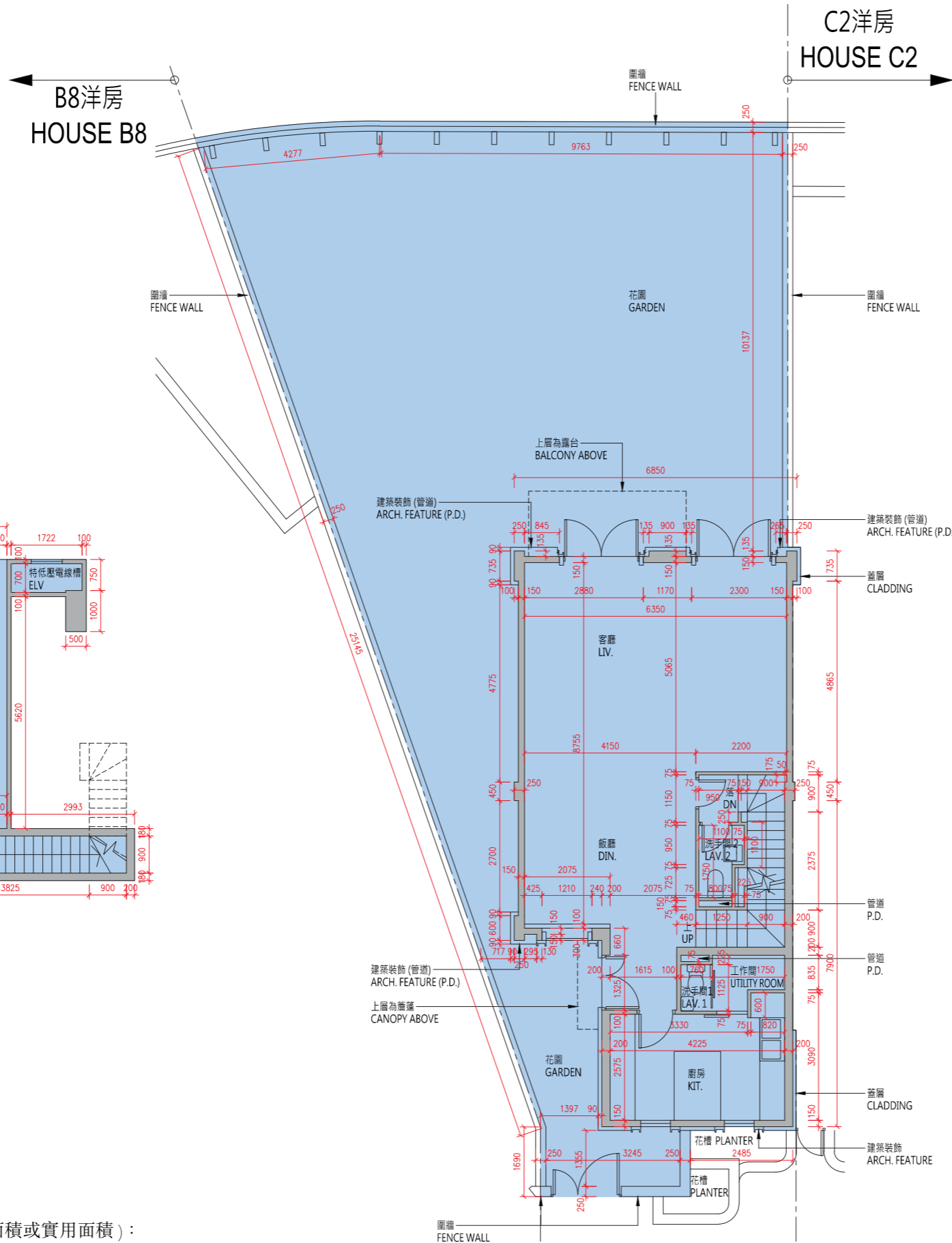
地庫1樓平面圖 B1/F Floor Plan
