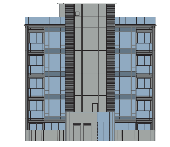
立面圖 B ELEVATION PLAN B
