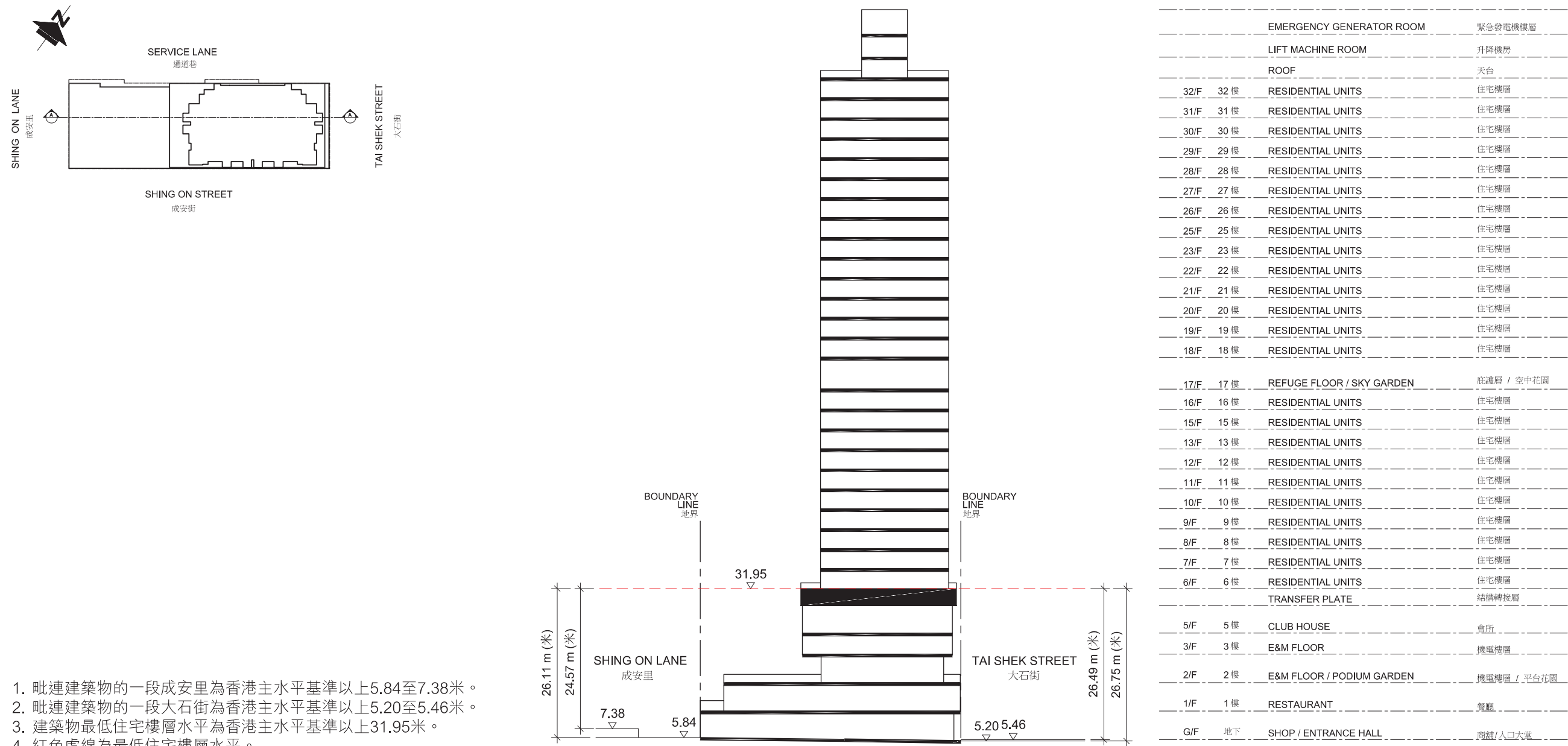
橫截面圖 A-A Cross - Section Plan A-A
