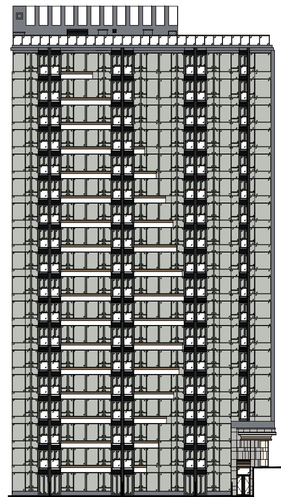
第3座 立面圖 TOWER 3 - ELEVATION PLAN
