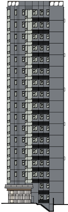
立面圖 5 ELEVATION PLAN 5
