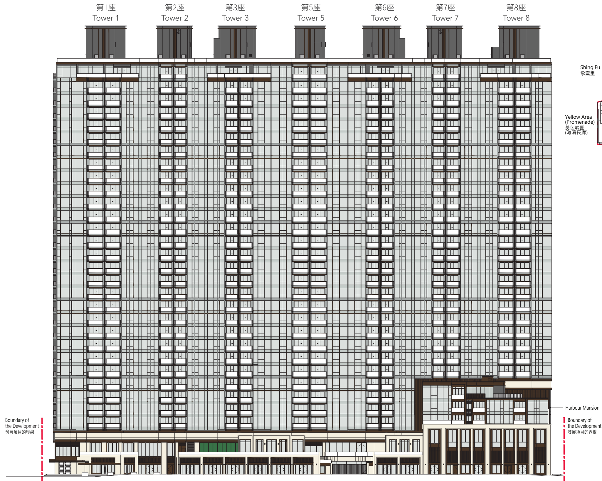
立面圖 1 Elevation 1
