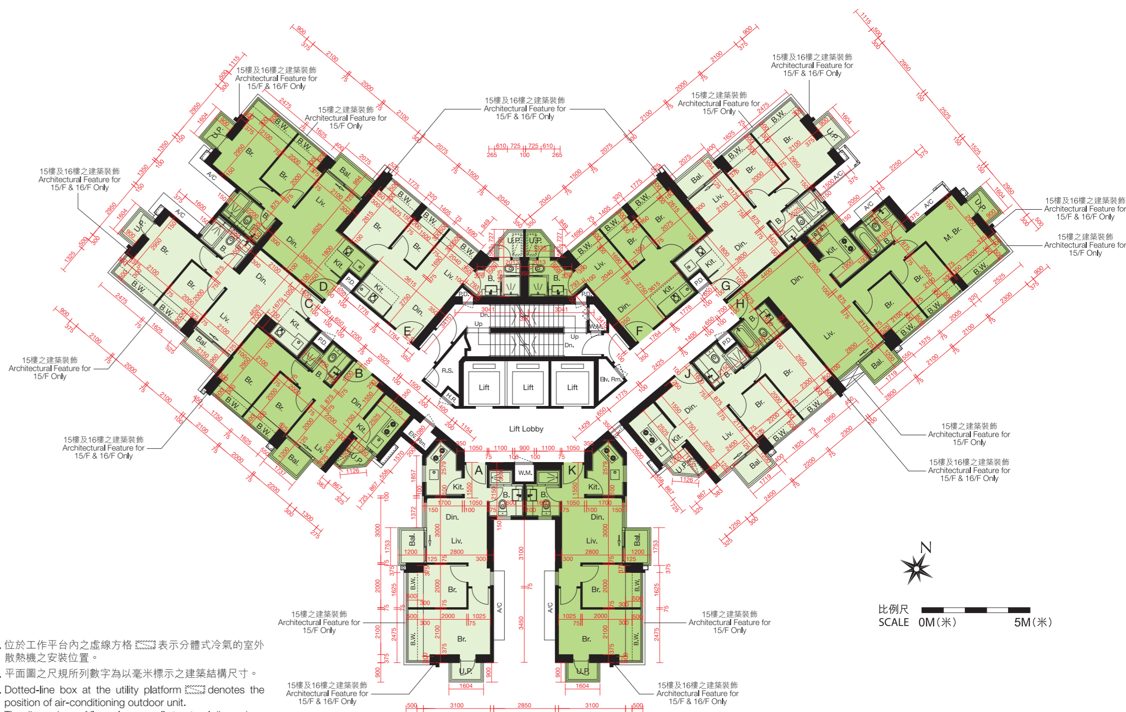
二樓至十六樓平面圖 2ND - 16TH FLOOR PLAN
