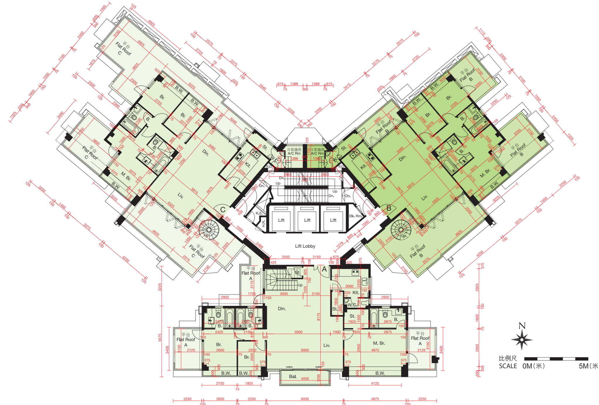
二十八樓平面圖 28TH FLOOR PLAN
