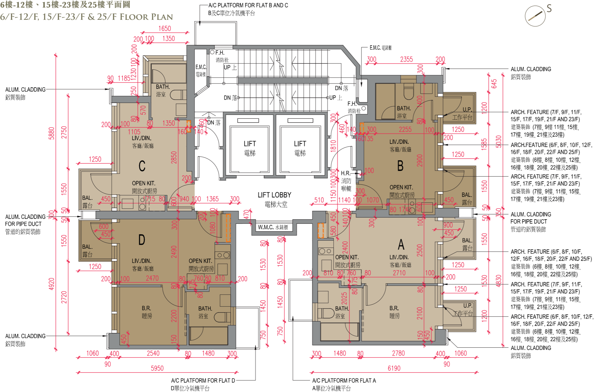
6樓-12樓、15樓-23樓及25樓平面圖
