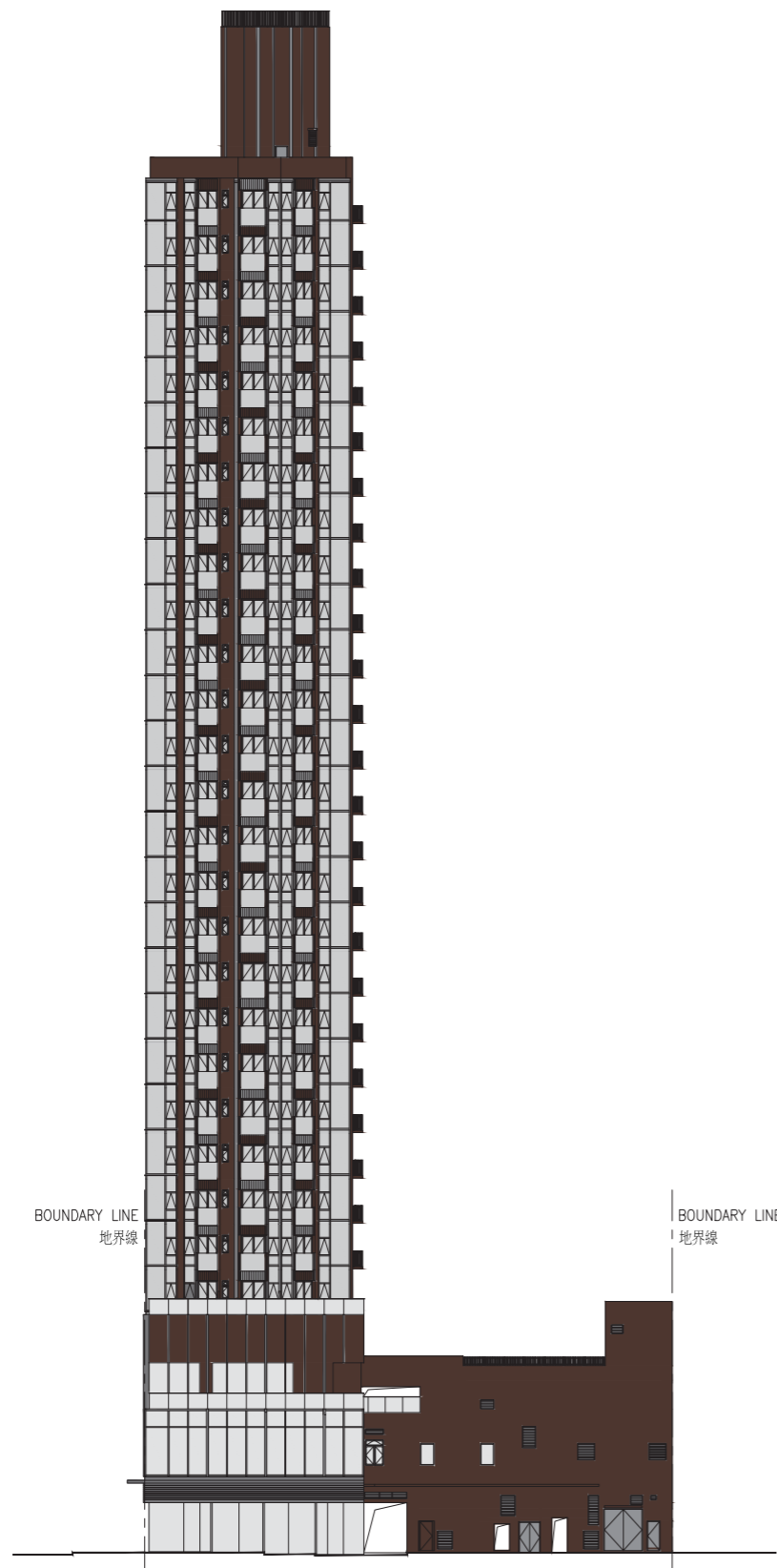
Southeast Elevation 東南立面圖
